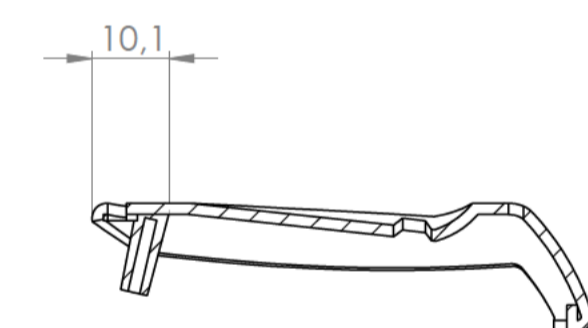
Sección / Section R-R
