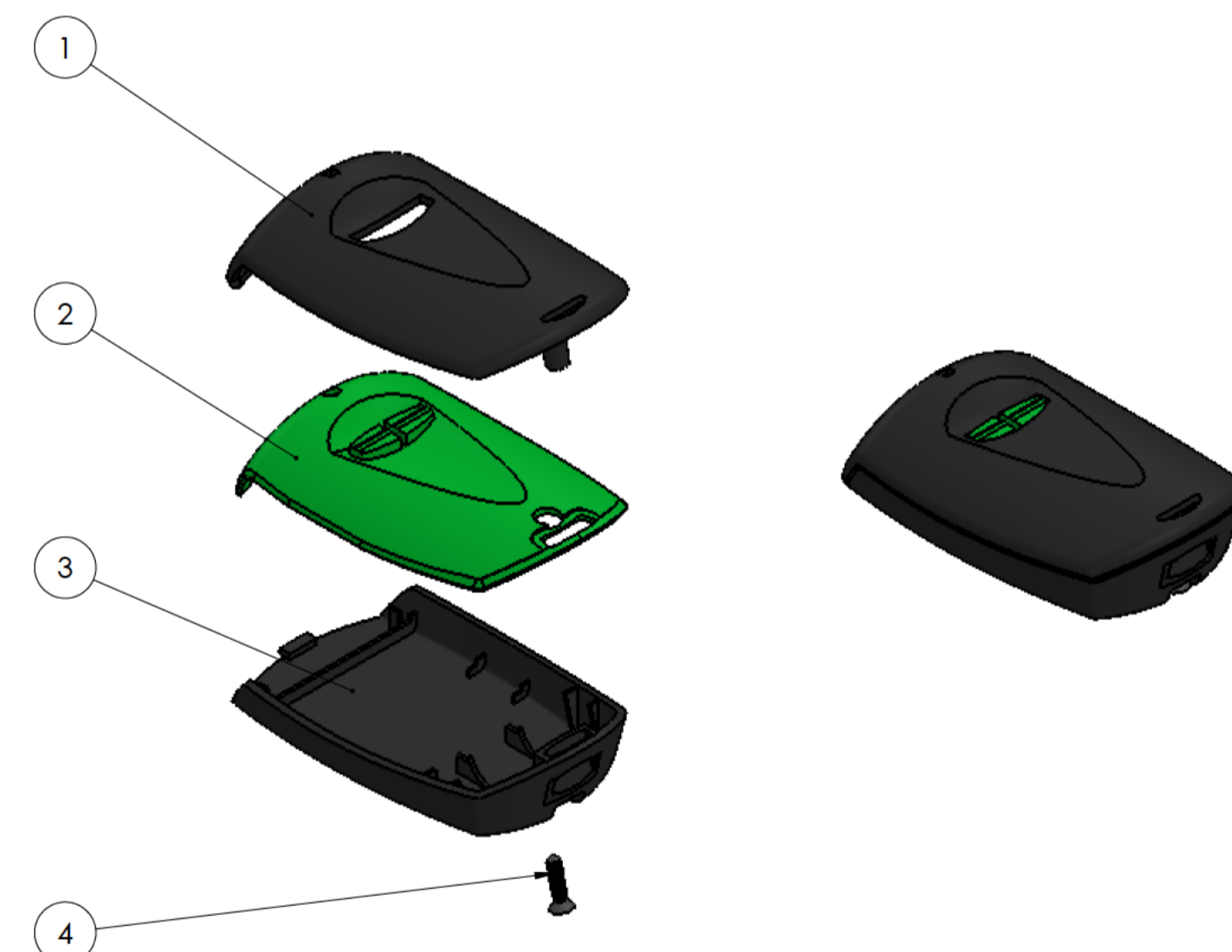
Conjunto Assembly
