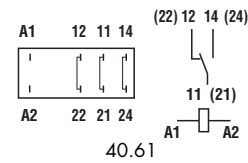
Ansicht auf die Anschlüsse
